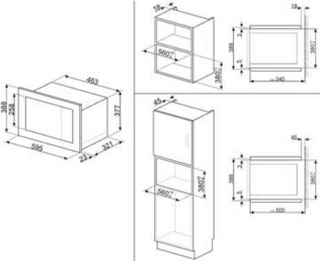
installazione a pensile o a colonna FMI020X
