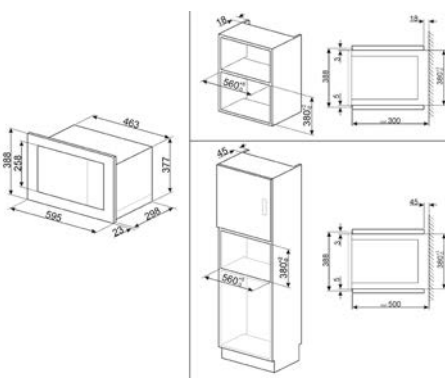
installazione a pensile o a colonna FMI017X
