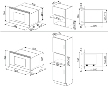
installazione a pensile o a colonna MP422, MP722, MP822
